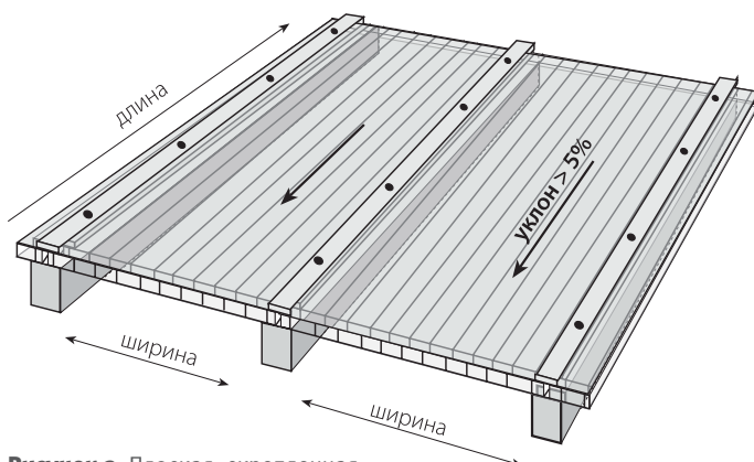
Рисунок 2. Плоская, скрепленная с двух сторон кровля.
