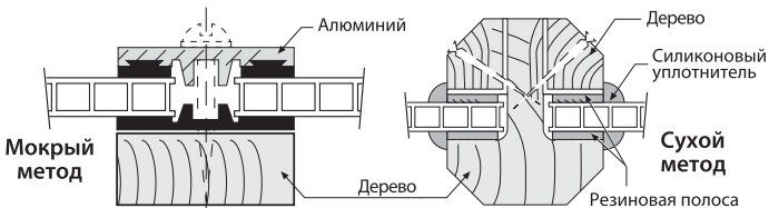
Рисунок 10. Деревянные соединительные профили.
